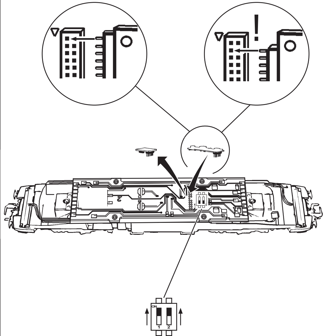
Dip-Schalter für Analogmodell / Dip-Switch for analouge model / Commutateur DIP pour modèle analogique
